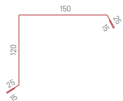
Závětrná lišta boční F02
